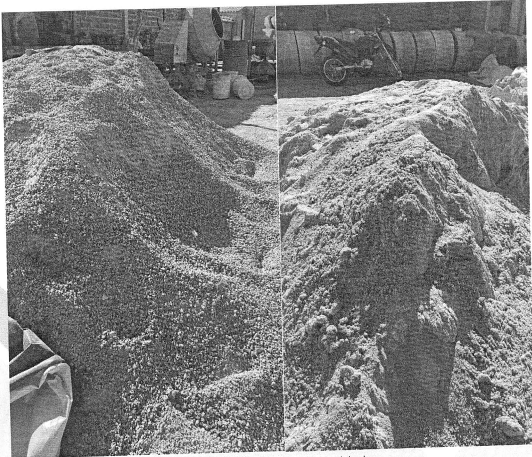
Foto 4- Agregados em estoque para produção de pré-moldados.
