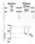
Detalhe Corrimão - DIMENSÕES
