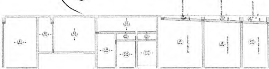
Armação positiva das lajes do pavimento 2. Superior (Eixo Y)
