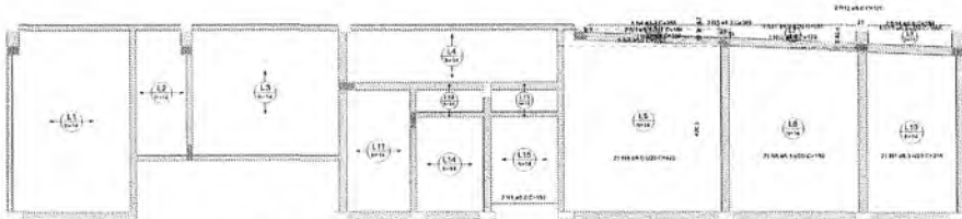
Armação positiva das lajes do pavimento 2. Superior (Eixo X)
