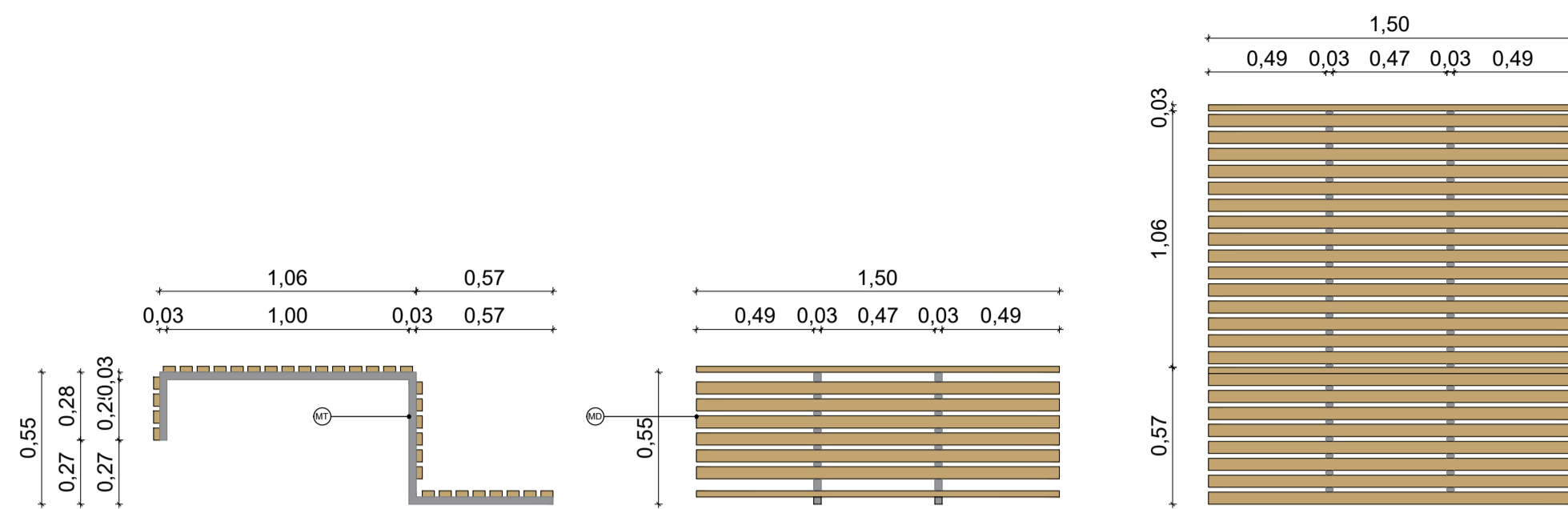
VISTA LATERAL BANCO T1 ESCALA: 1/25
