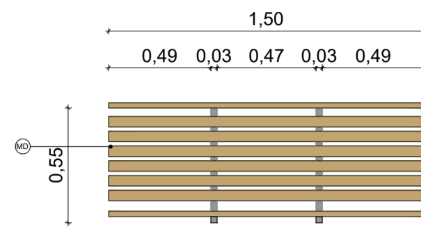
VISTA FRONTAL BANCO T2 ESCALA: 1/25
