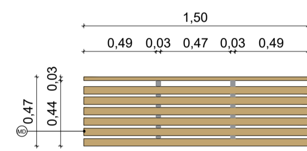
VISTA FRONTAL BANCO T3 ESCALA: 1/25
