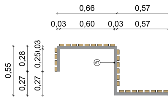
VISTA LATERAL BANCO T2 ESCALA: 1/25
