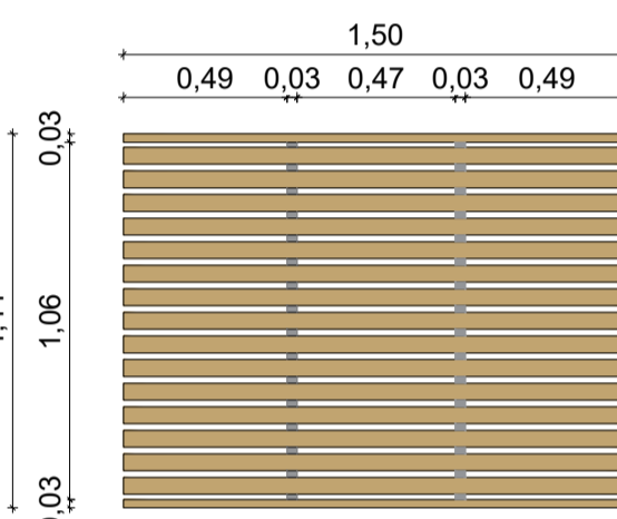
VISTA SUPERIOR BANCO T3 ESCALA: 1/25
