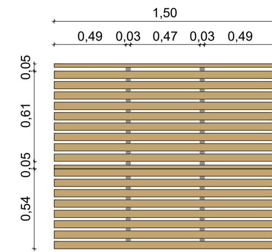
VISTA SUPERIOR BANCO T2 ESCALA: 1/25
