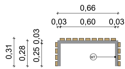
VISTA LATERAL BANCO T4 ESCALA: 1/25
