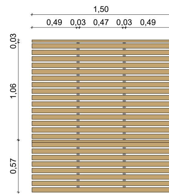
VISTA SUPERIOR BANCO T1 ESCALA: 1/25
