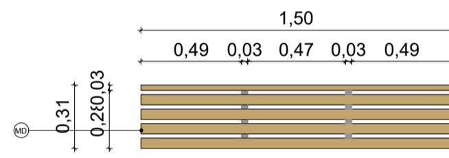
VISTA FRONTAL BANCO T4 ESCALA: 1/25
