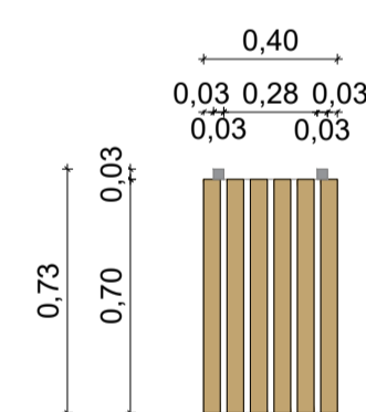
VISTA FRONTAL LIXEIRA L1 ESCALA: 1/25
