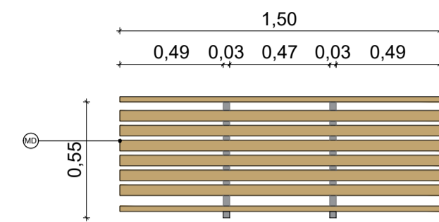
VISTA FRONTAL BANCO T1 ESCALA: 1/25
