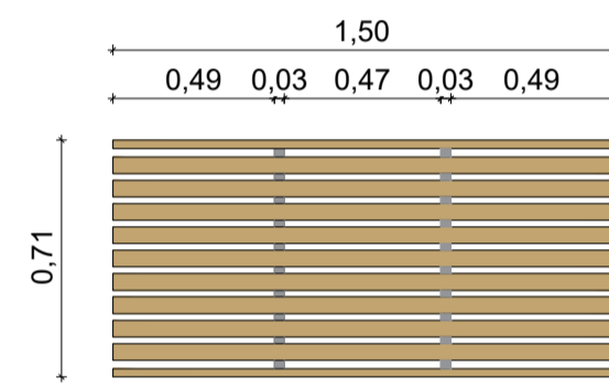
VISTA SUPERIOR BANCO T4 ESCALA: 1/25
