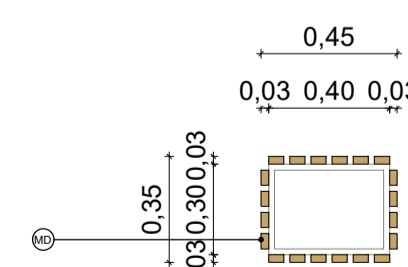
VISTA SUPERIOR LIXEIRA L2 ESCALA: 1/25
