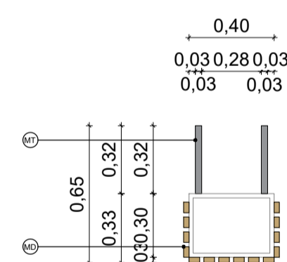
VISTA SUPERIOR LIXEIRA L1 ESCALA: 1/25
