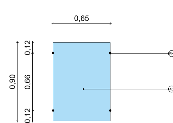
EXPOSITOR DE CARTAZ A1 - VISTA FRONTAL ESCALA: 1/25
