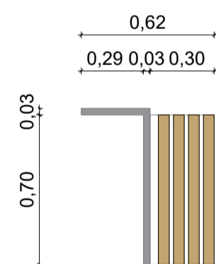
VISTA LATERAL LIXEIRA L1 ESCALA: 1/25
