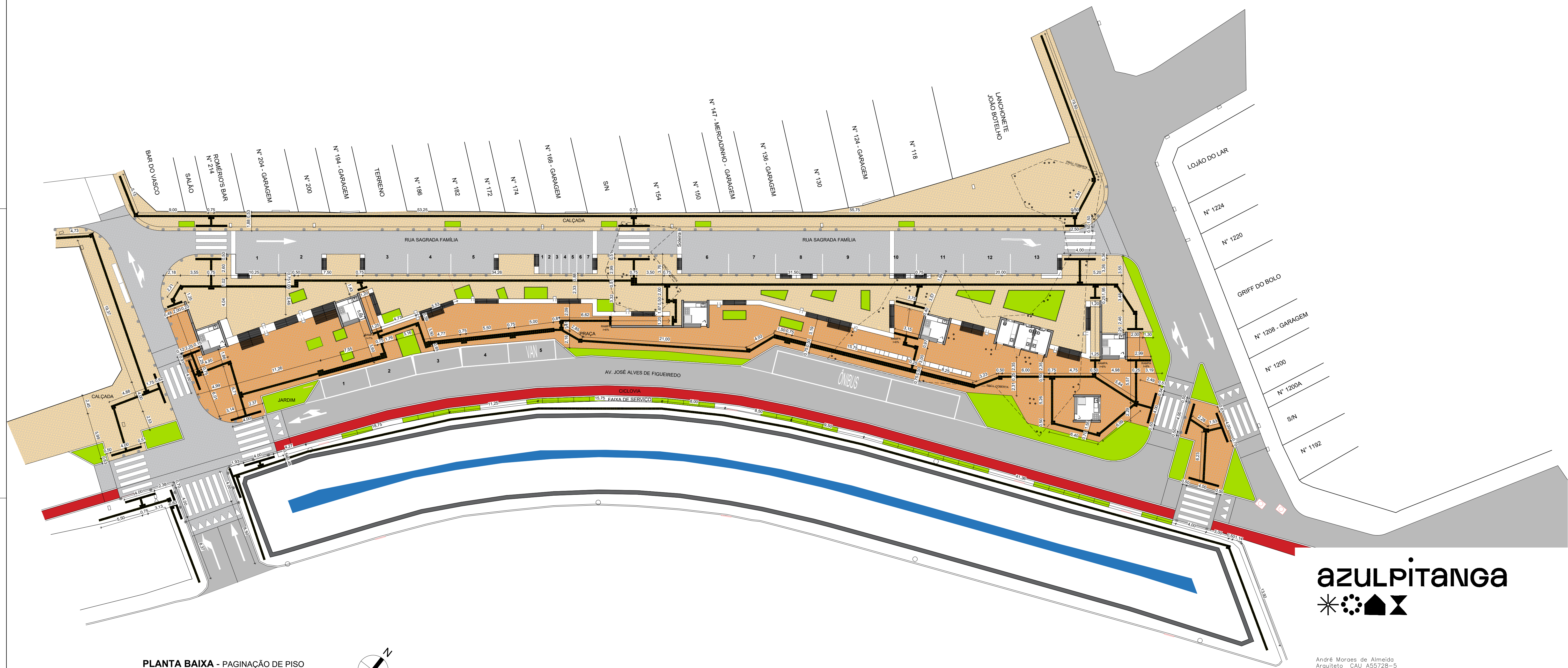
PLANTA BAIXA - PAGINAÇÃO DE PISO E ACESSIBILIDADE ESCALA: 1/250
