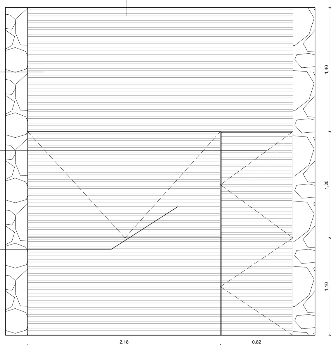
FACHADA 01 ESCALA: 1/25
