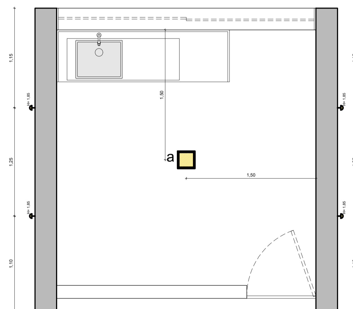
PLANTA DE ILUMINAÇÃO ESCALA: 1/25
