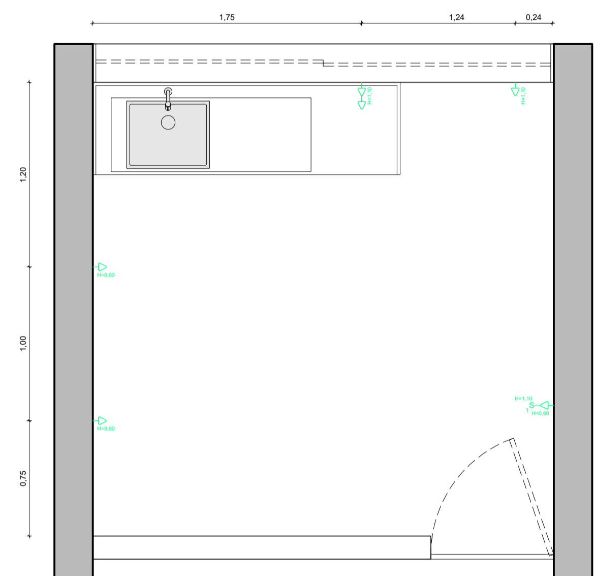
PLANTA DE PONTOS ELÉTRICOS ESCALA: 1/25
