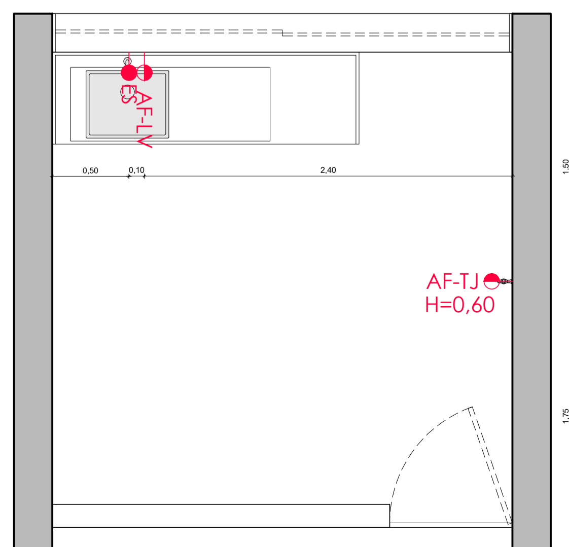
PLANTA DE PONTOS HIDRÁULICOS ESCALA: 1/25
