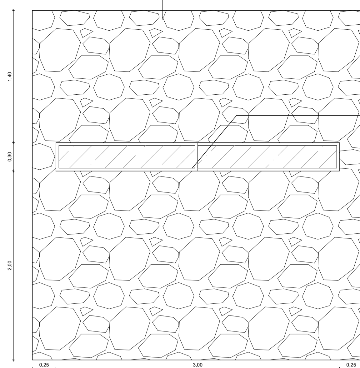
FACHADA 03 ESCALA: 1/25
