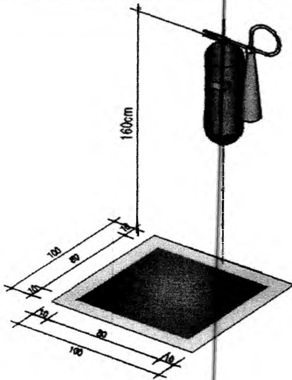
Imagem 01. Representação do extintor instalado e sinalizado
