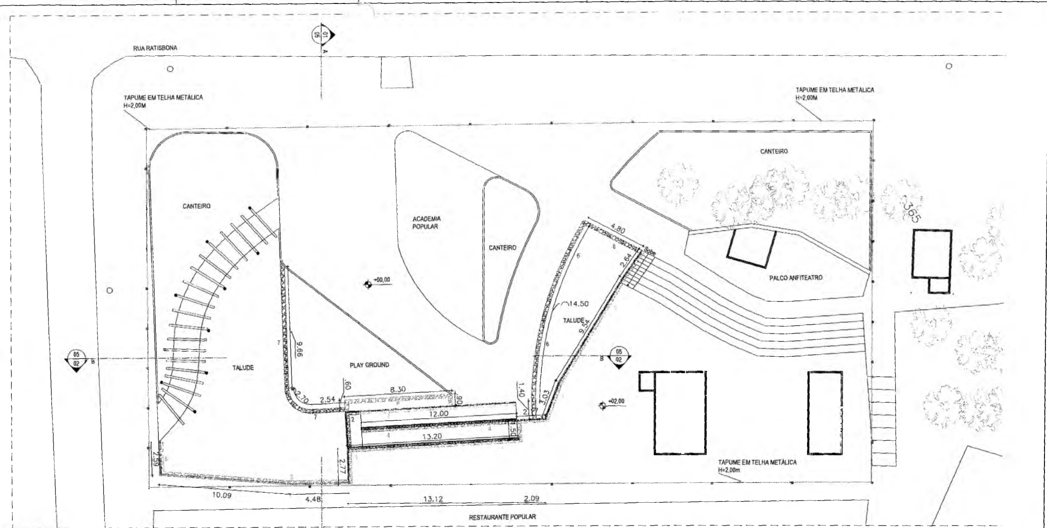
01 PLANTA LOCAÇÃO ALVENARIA DE PEDRA ARGAMASSADA ESC. 1/725
