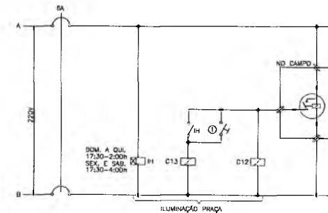
DIAGRAMA DE COMANDO QD-01D (MEDIÇÃO 01D)
