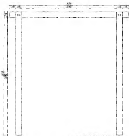
04 VISTA FRONTAL PERGOLADO
