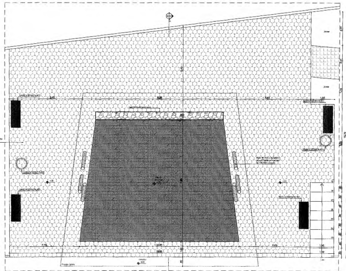
02 AMPLIAÇÃO PALCO
