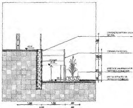
02 CORTE AA RAMPA
