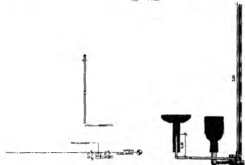
04 CORTE WC-04 1:20
