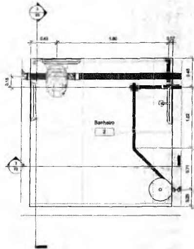
1 Planta Baixa Banheiro 2 1:20
