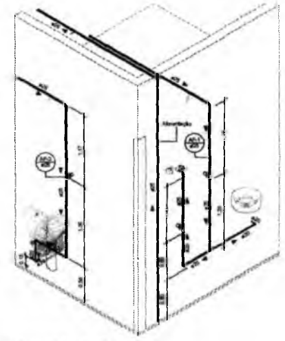
2 Isometrico Banheiro 01
