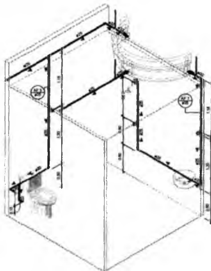
4 Isometrico Banheiro 02
