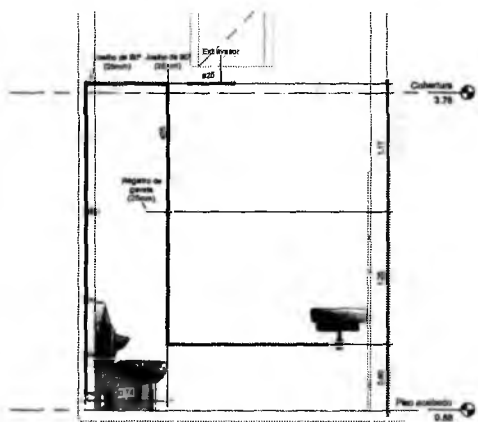
3 4- Corte 02 Banheiro 04 1:20
