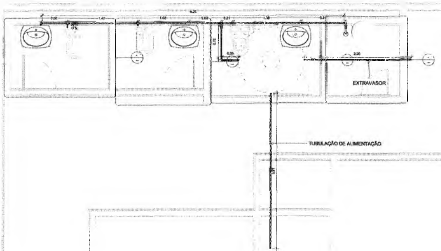
Planta Baixa - ÁGUA FRIA 1:20
