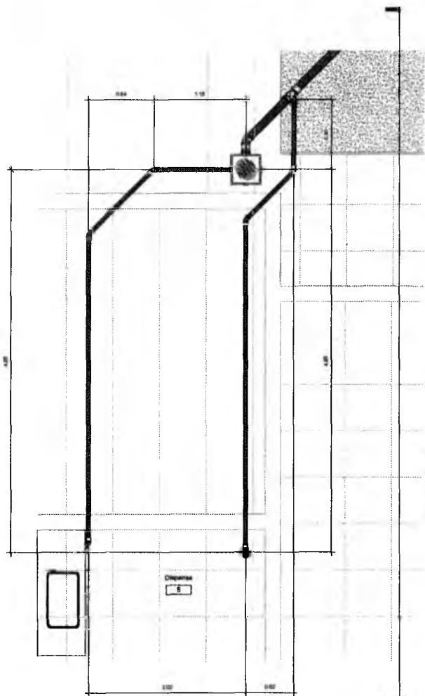
1 Planta Baixa Dispensa 5 1:20
