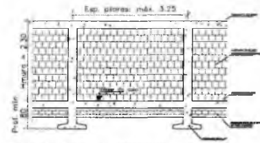
DETALHE MURO DE CONTORNO ESC. 1/50
