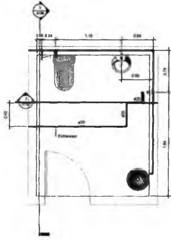
1 Planta Baixa Banheiro 04 1:20
