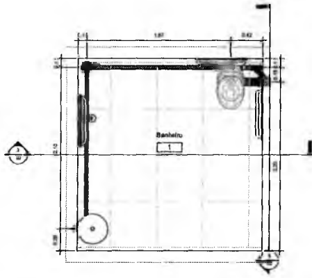
1 Planta Baixa Banheiro 1 1:20
