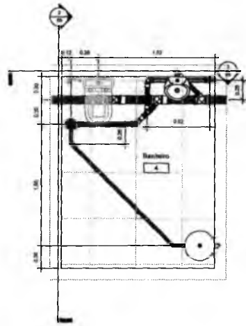
1 Planta Baixa Banheiro 4 1:20
