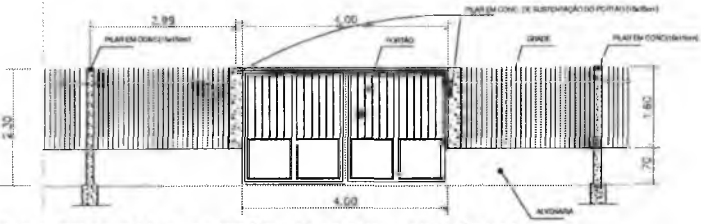
MURO FRONTAL E PORTÃO - VISTA ESQUEMÁTICA ESC. 1/50
