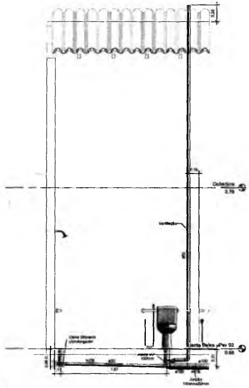
2 01 - Corte 01 Banheiro 01 1:20
