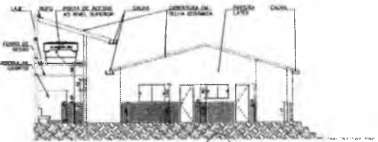
CORTE B-B ESC. 1/100
