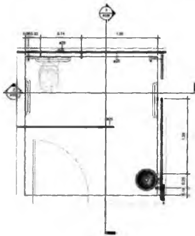
1 Planta Baixa Banheiro 02 1:20
