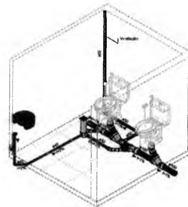
4 Isométrico Banheiro 3
