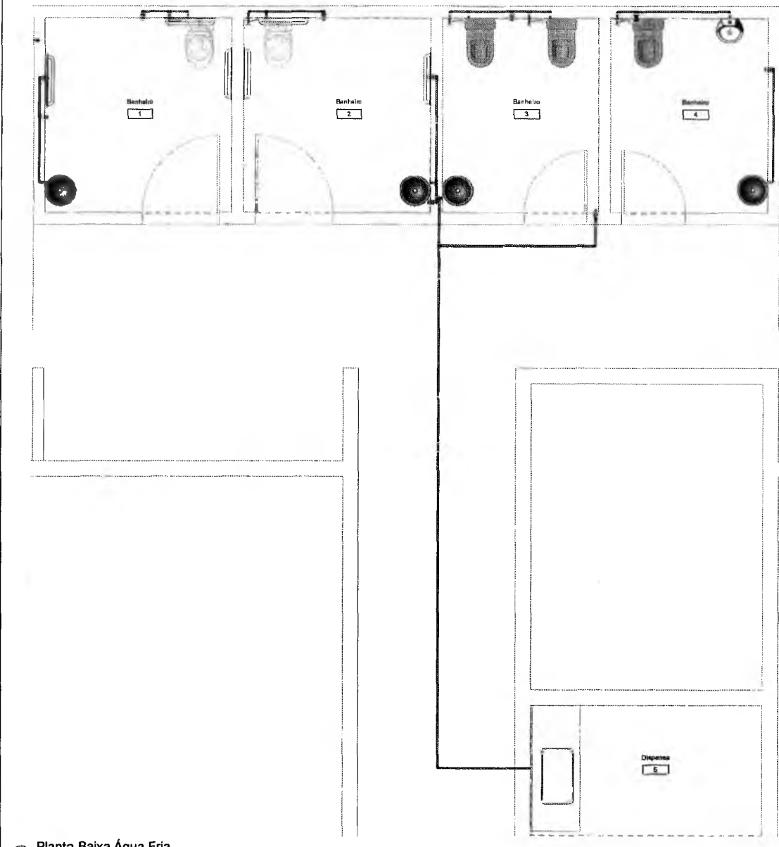
1 Planta Baixa Água Fria 1:20
