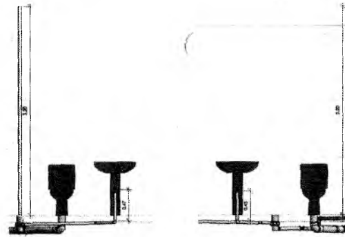
02 CORTE WC-01.1 1:20
