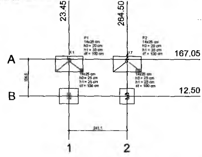
Planta de locação escala 1:50
