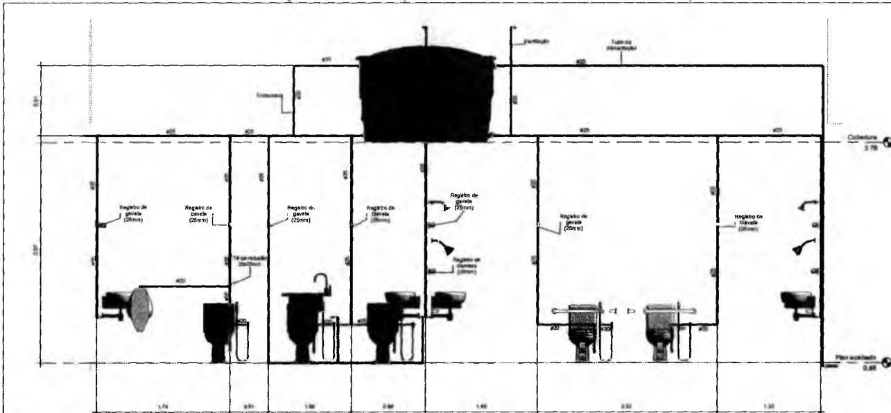
③ 6 - Corte 02 Reservatório 1:20
