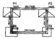
Forma do pavimento FUNDAÇÃO escala 1:50
