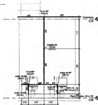
5 Isométrico Banheiro 03
