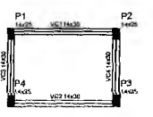
Forma do pavimento CAIXA escala 1:50
