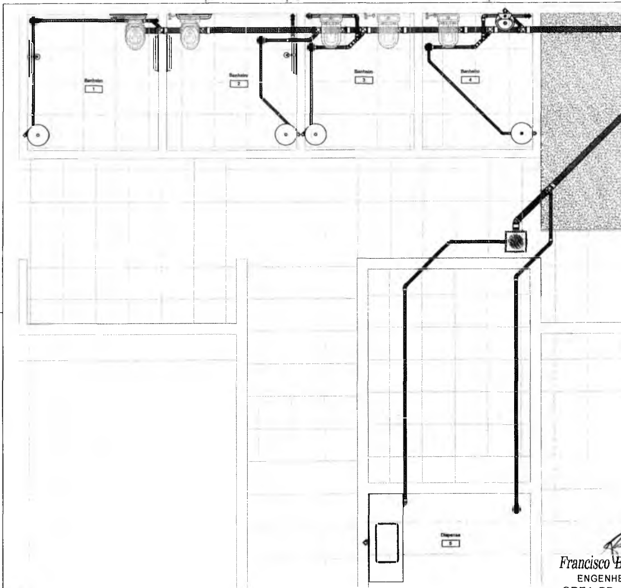
1 Planta Baixa Sanitário 1:20
