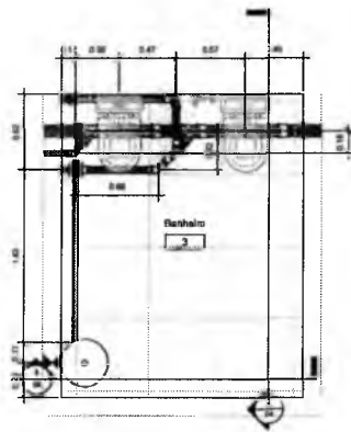
1 Planta Baixa Banheiro 3 1 : 20
