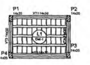
Forma do pavimento TÉRREO escala 1:50
