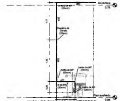
4 1- Corte 02 Banheiro 01 1:20
