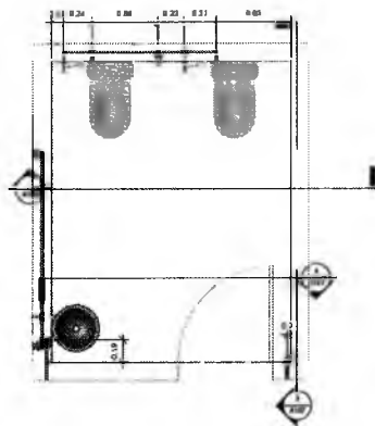
1 Planta Baixa Banheiro 03 1:20
