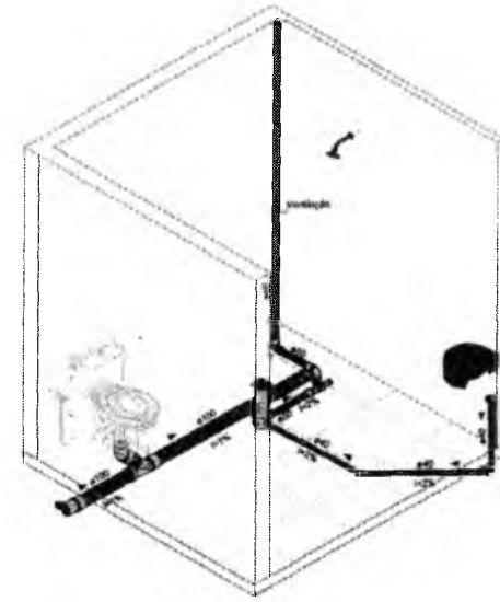
4 Isométrico Banheiro 2
