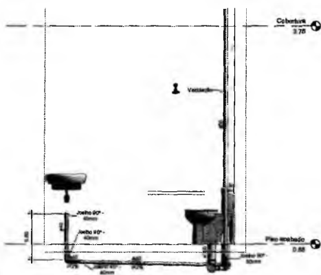
3 01 - Corte 02 Banheiro 01 1:20
