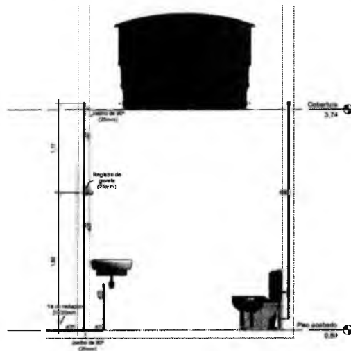
3- Corte 02 Banheiro 3 1:20
