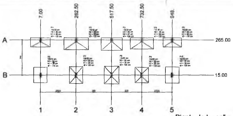
Planta de localização
