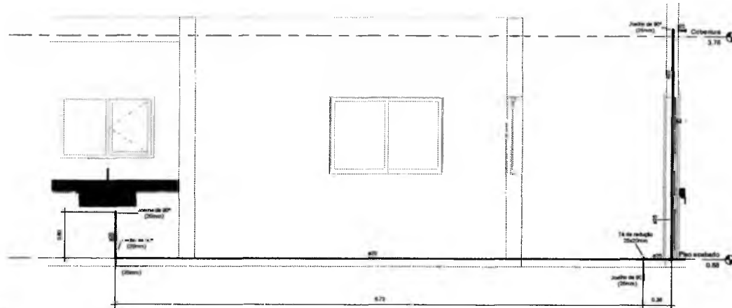
2 5- Corte 01 Dispensa 1:20
