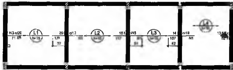
Armação negativa das lajes do pavimento TÉRREO (Eixo X)
