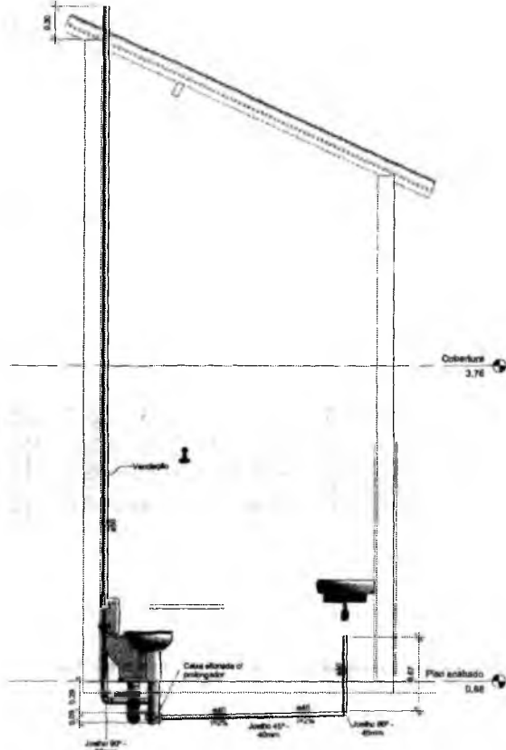
3 02 - Corte 02 Banheiro 02 1:20
