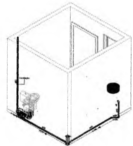
4 Isométrico Banheiro 1
