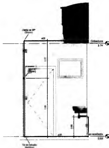
4 3- Corte 03 Banheiro 03 1:20
