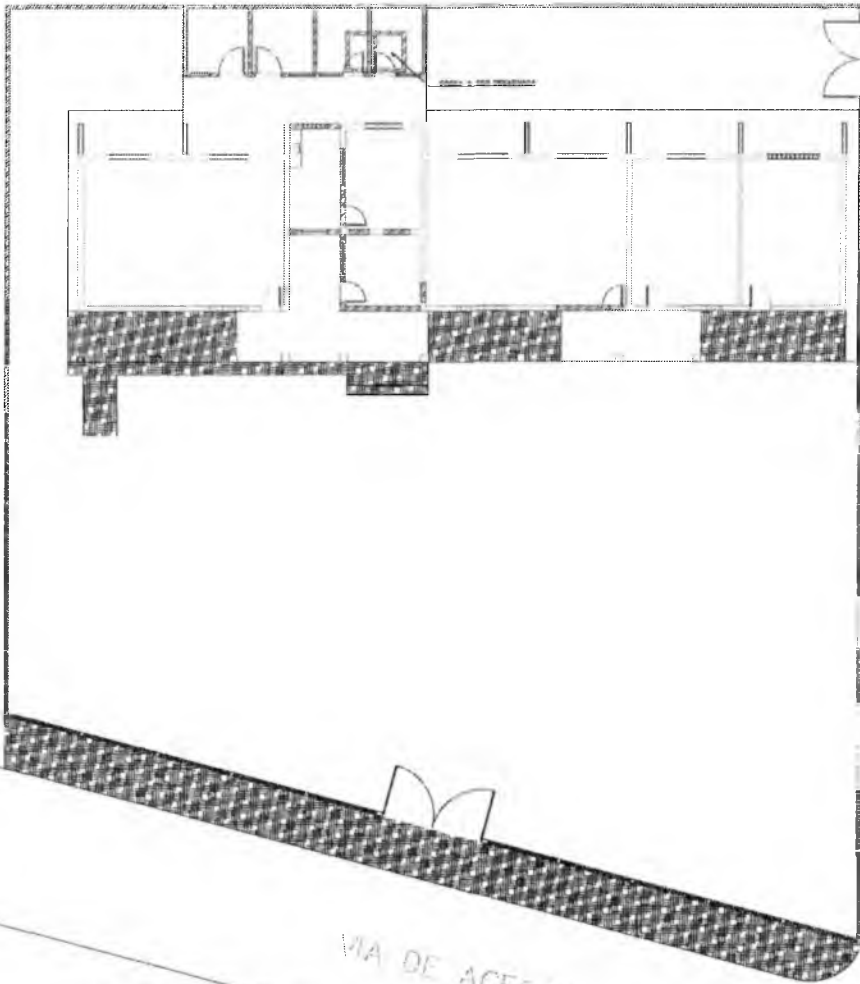
PLANTA GERAL ESC. 1/100
