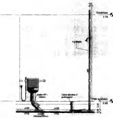
2 02 - Corte 01 Banheiro 02 1:20
