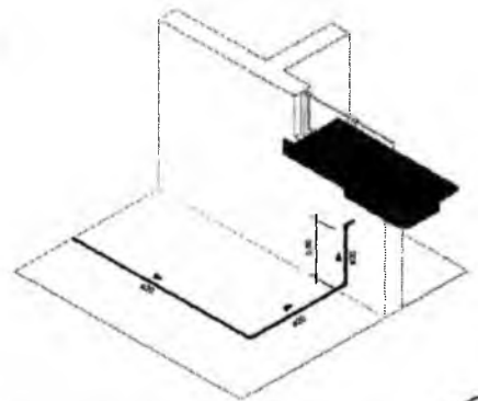
① isométrico Dispensa
