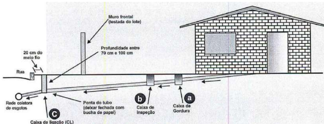
FIGURA 8. CROQUI DE LIGAÇÃO PREDIAL DE ESGOTO (ORIENTATIVO).
