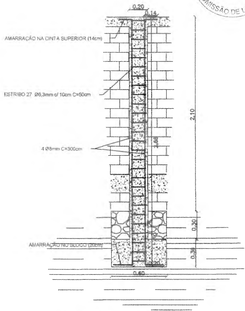
ARMADURA DO PILAR esc 1:25
