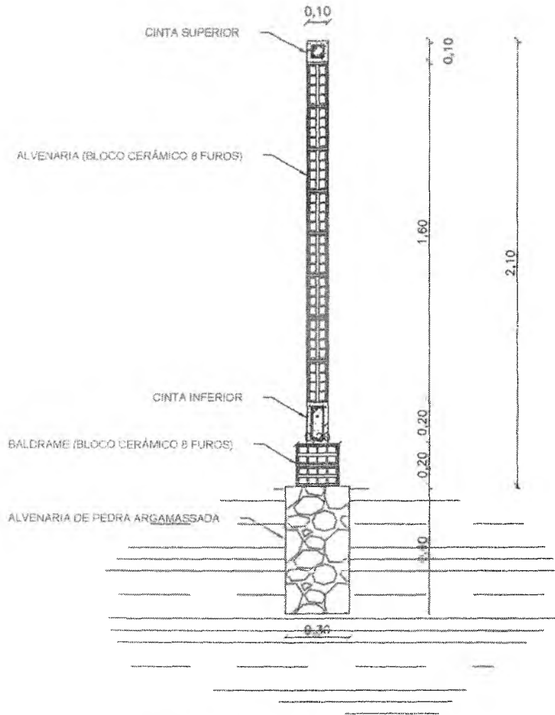
CORTE TRANSVERAL DO MURO esc 1:25
