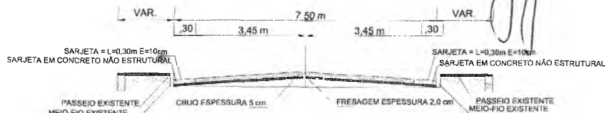
PERFIL TRANSV. SEM ESCALA
