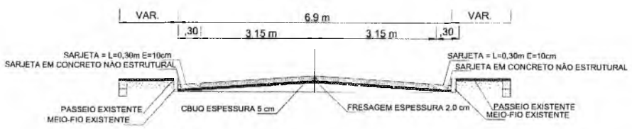
PERFIL TRANSV. SEM ESCALA
