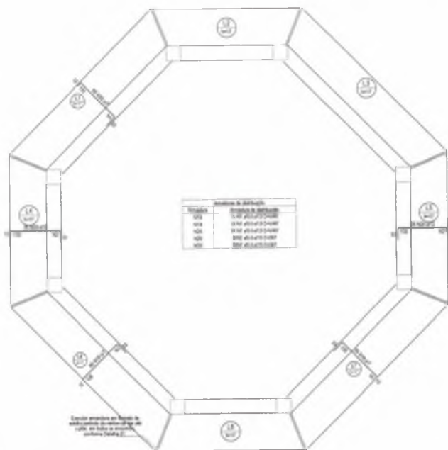
Armação negativa das lajes do pavimento SUPERIOR (Eixo X)
