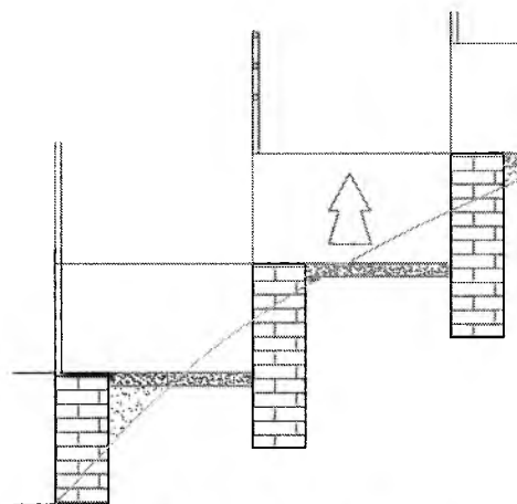
05 | DET. ESCADA ESC 1/100
