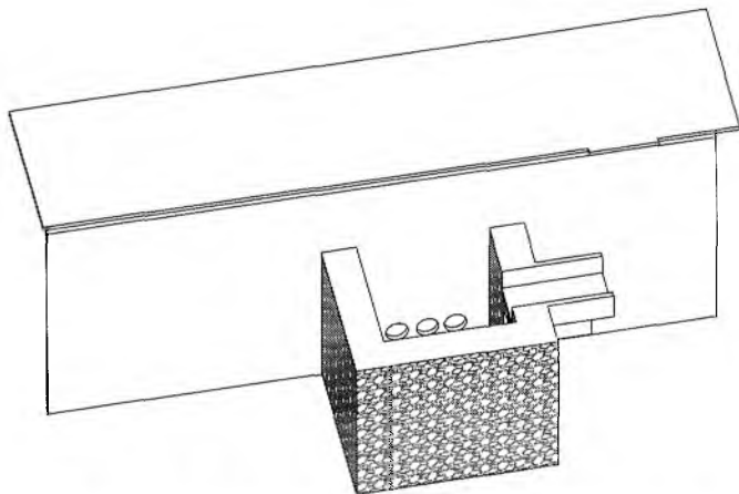
DETALHE DA CAIXA DE DRENAGEM - PERSPECTIVA 3
