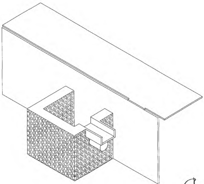
DETALHE DA CAIXA DE DRENAGEM - PERSPECTIVA 1
