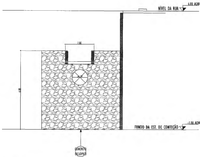
DETALHE DA CAIXA DE DRENAGEM - CORTE AA
