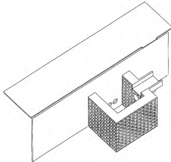
DETALHE DA CAIXA DE DRENAGEM - PERSPECTIVA 2
