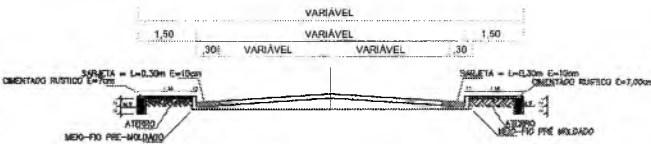
PERFIL TRANSV. SEM ESCALA
