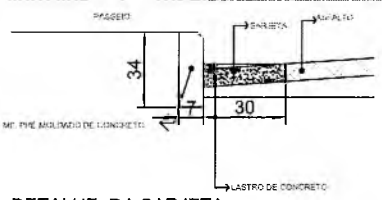
DETALHE DA SARJETA ESCALA - SEM ESCALA
